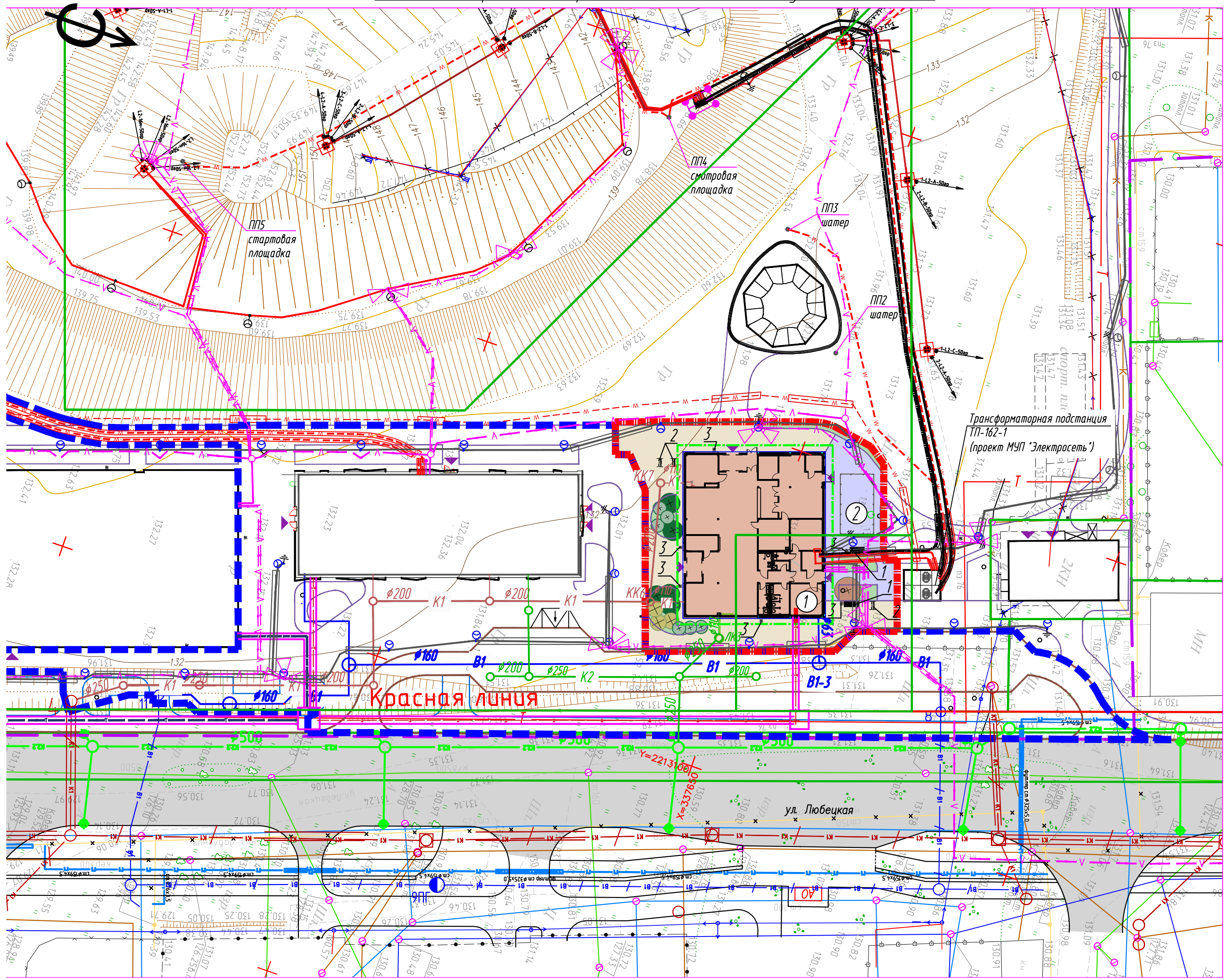
Схема планировочной организации земельного участка. М 1:500
